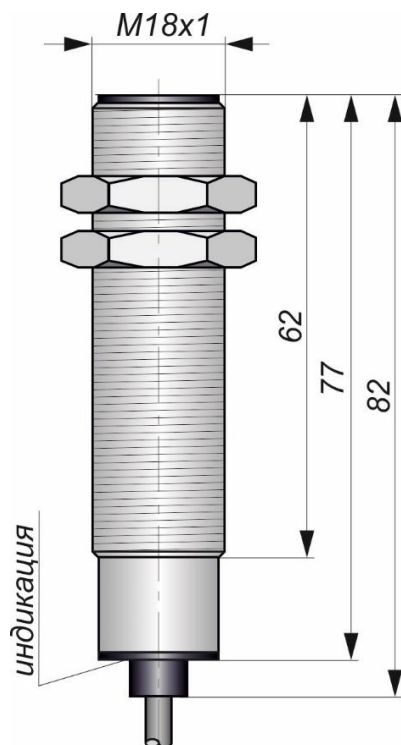
Габаритный чертеж
